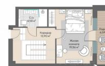
11 этаж
